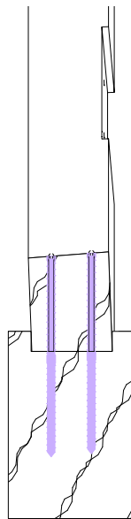
SECTION A-A M1:5
